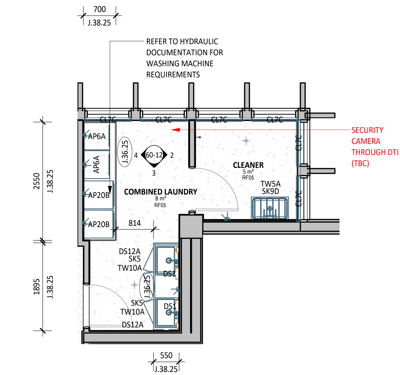
1 PLAN DETAIL 1 : 50
